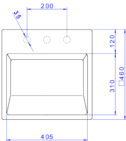
Desenho Técnico
